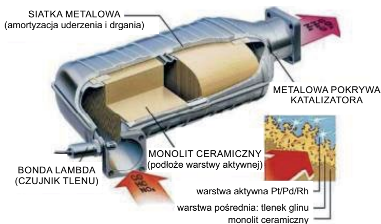
Rys. 1. Schemat budowy katalizatora trójfunkcyjnego
