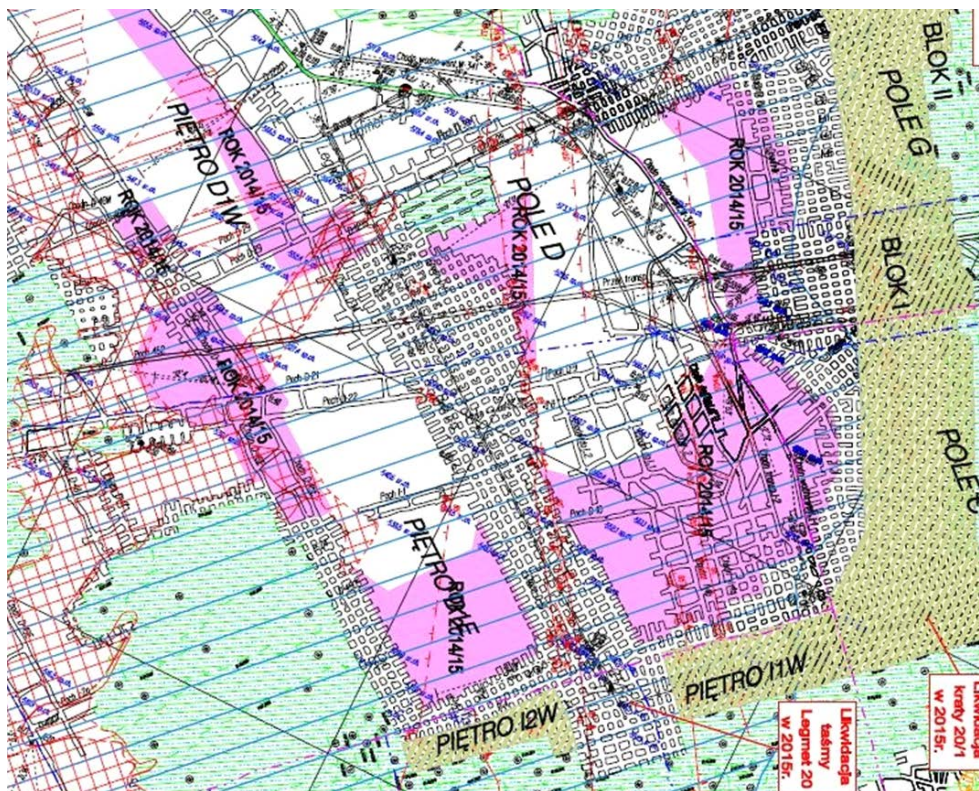
Rys. 1. Szkic wyrobisk górniczych w oddziale G-23 w kopalni Polkowice-Sieroszowice stan na lata 2014–2015 (według Działu Tapań Kopalni Polkowice-Sieroszowice) znaczenie kolorów na rysunku: różowy oznacza rozcinkę w latach 2014–2015, oliwkowy oznacza likwidację w latach 2014–2015
