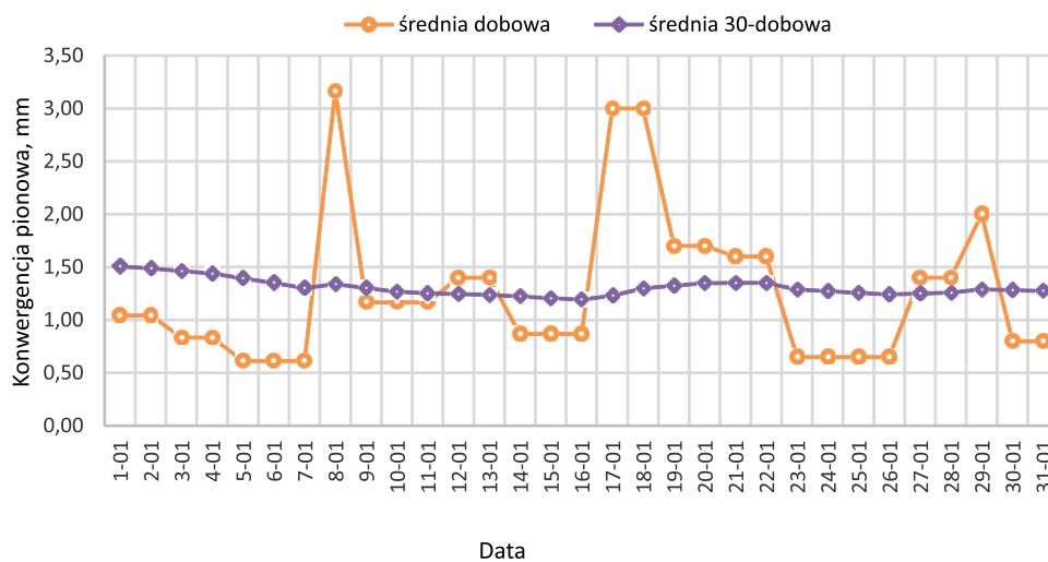
Rys. 4. Średnia dobowa pionowej konwergencji na tle średniej 30-dobowej w styczniu 2016 roku oddział G-23 (wg Markowiak 2017)
