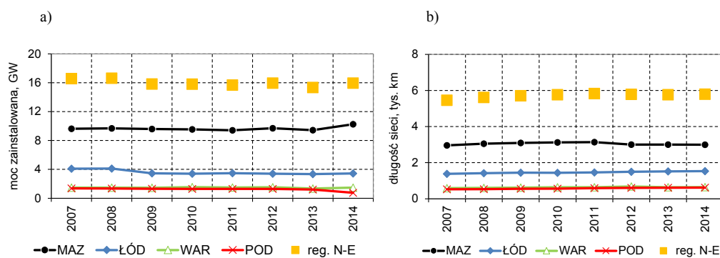
Rys. 7. Potencjał ciepłowniczy w regionie N-E wg zainstalowanej mocy (a) i długości sieci ciepłowniczej (b) Źródło: opracowanie własne na podst. (URE – Energetyka cieplna... 2008–2015)
