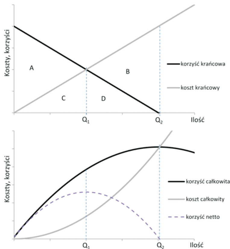
Rys. 3. Reguły decyzyjne
