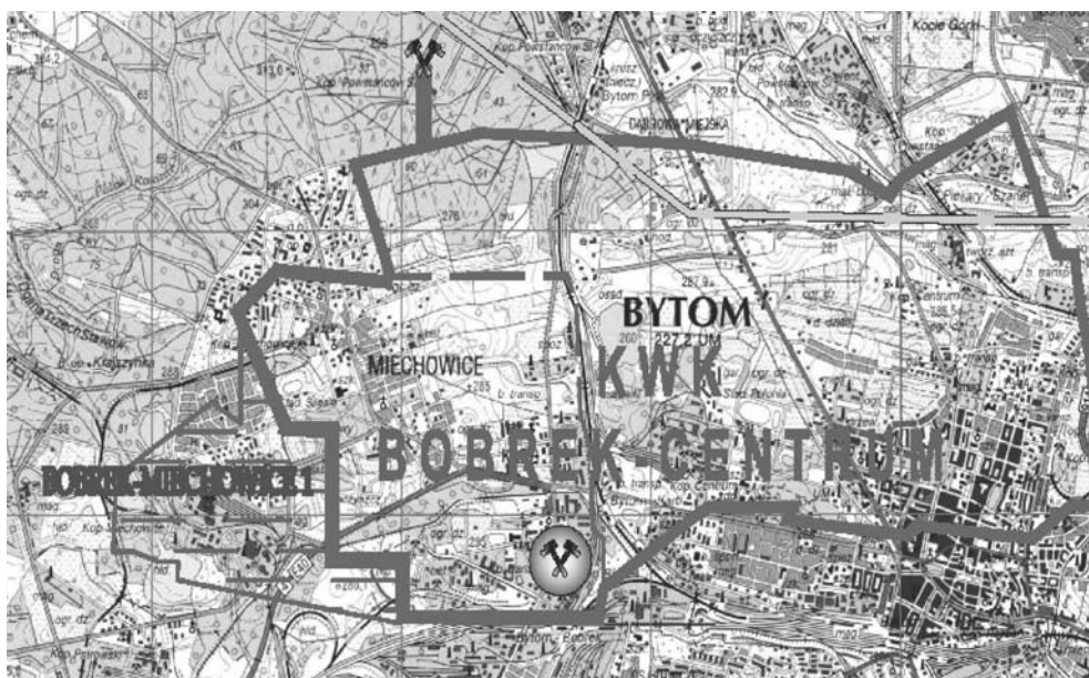
Rys. 6. Położenie złoża „Bobrek-Miechowice I”
