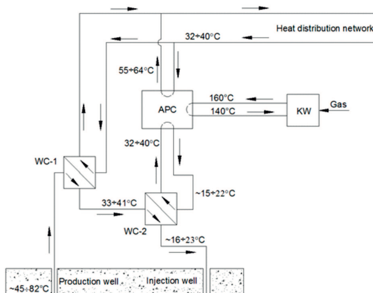
Rys. 2. Uproszczony schemat kaskadowego schładzania wód termalnych Fig. 2. The scheme of the thermal waters cascade cooling
