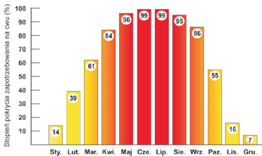
Rys. 4. Stopień pokrycia zapotrzebowania na wodę użytkową przez instalacja solarną w poszczególnych miesiącach roku w warunkach polskich (solar shop; www.solarshop.pl)
